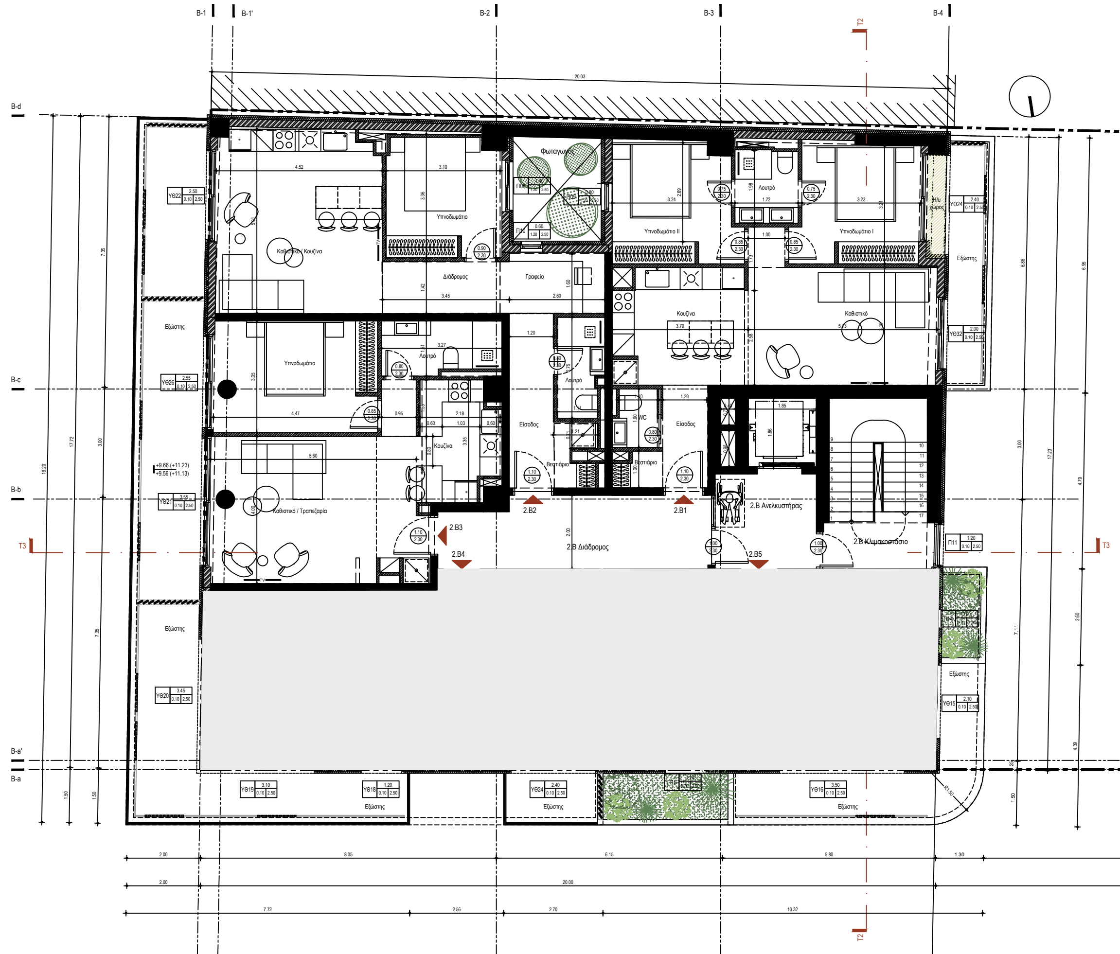
ΚΤΙΡΙΟ Β ΚΑΤΟΨΗ 3ου ΟΡΟΦΟΥ ΚΛΙΜΑΚΑ 1:100
