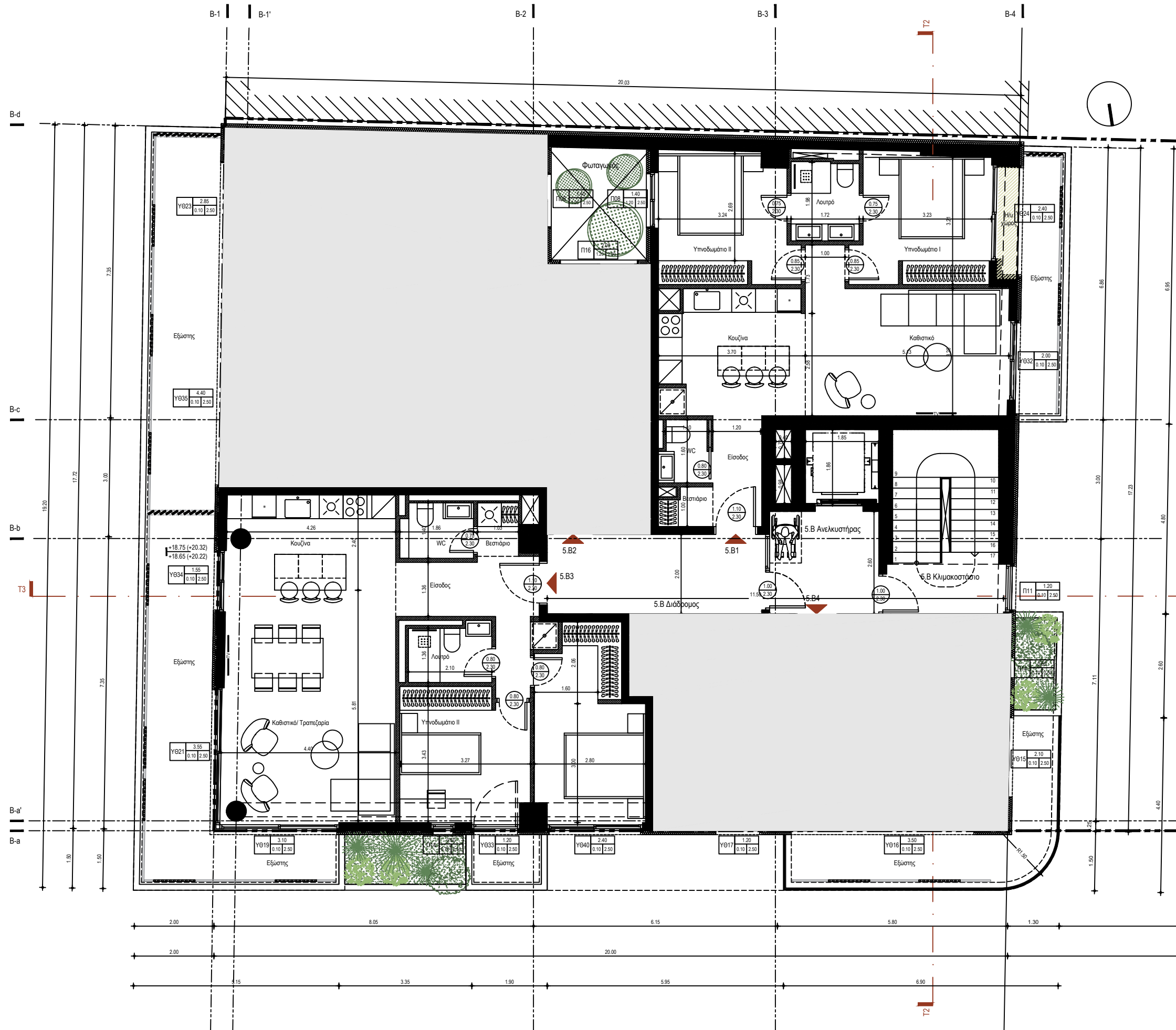
ΚΤΙΡΙΟ Β ΚΑΤΟΨΗ 6ου ΟΡΟΦΟΥ ΚΛΙΜΑΚΑ 1:100
