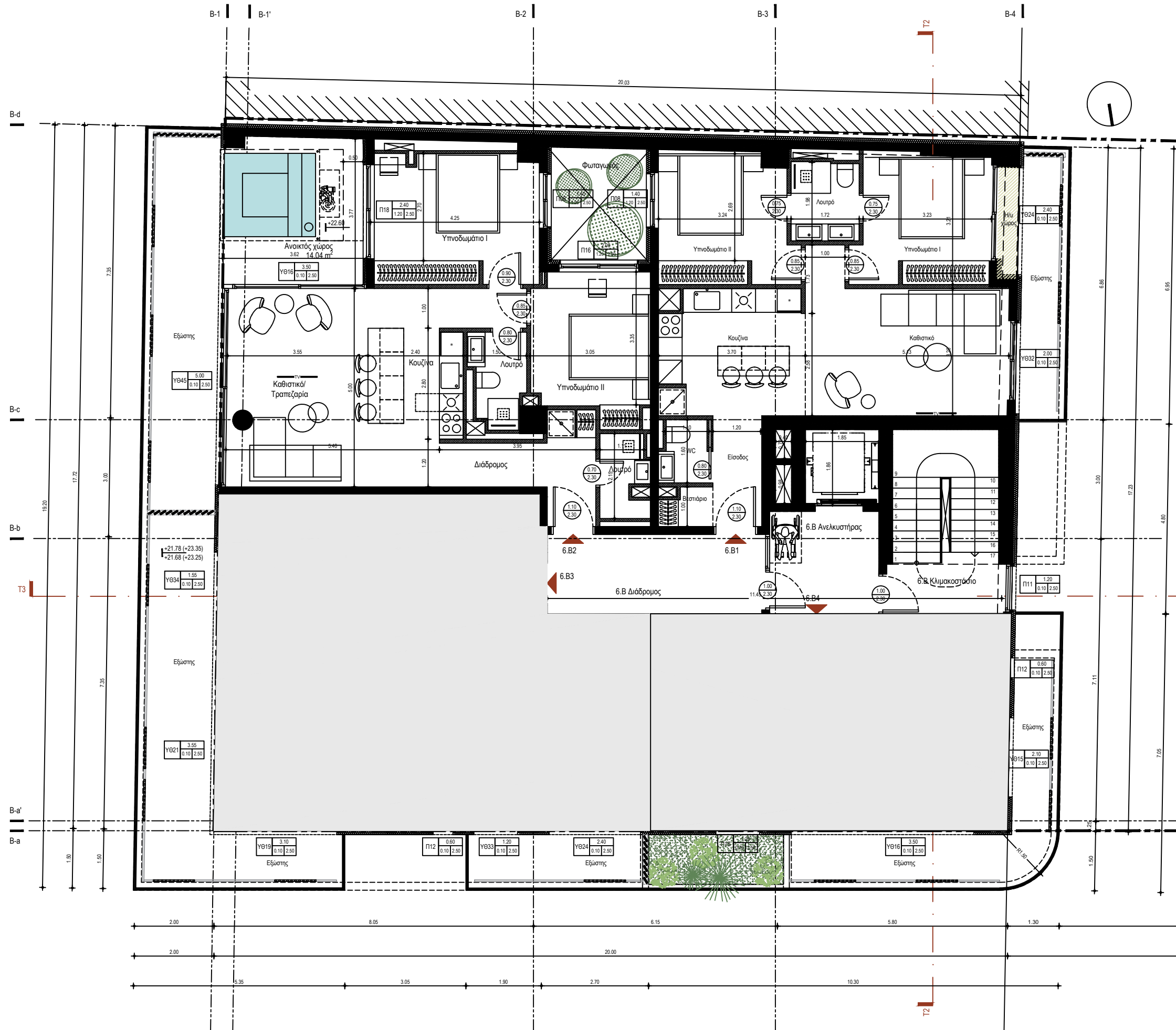
ΚΤΙΡΙΟ Β ΚΑΤΟΨΗ 7ου ΟΡΟΦΟΥ ΚΛΙΜΑΚΑ 1:100
