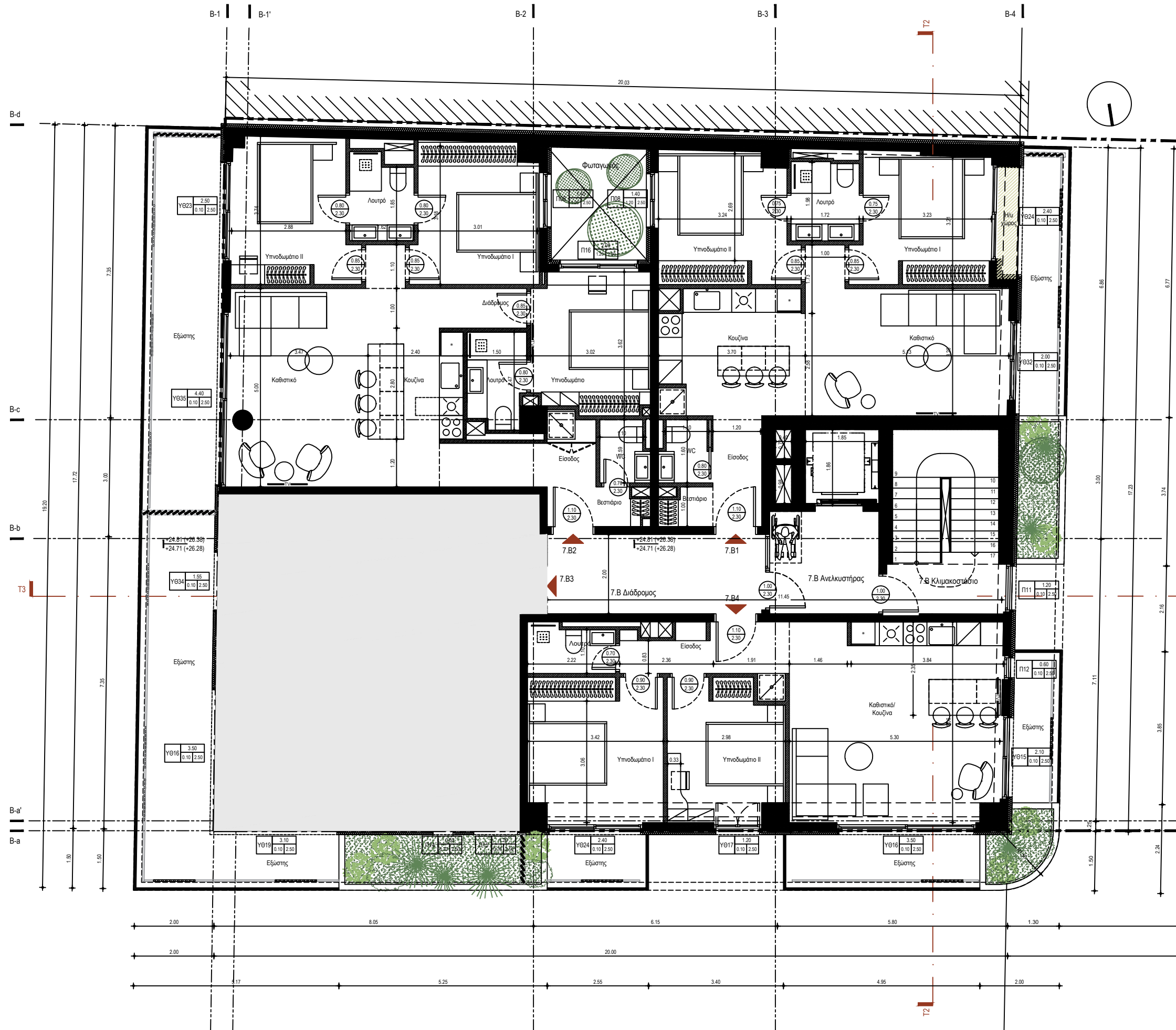
ΚΤΙΡΙΟ Β ΚΑΤΟΨΗ 8ου ΟΡΟΦΟΥ ΚΛΙΜΑΚΑ 1:100
